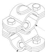
90300__ Bride à croix Kreuzbride
